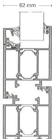
ADS 60 CH.HD - Ouverture intérieure Dormant classique et ouvrant, avec toile épaissie (2,8 mm)
